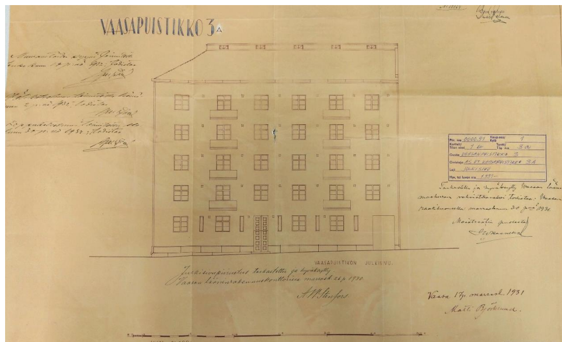
Kuva 23: Valokuva vuonna 1931 laaditusta julkisivupiirustuksesta Vaasanpuistikon suuntaan. Vaasan kaupungin rakennusvalvonta.
