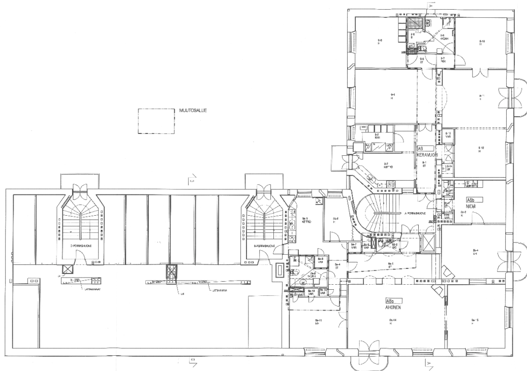
Kuva 33: Valokuva rakennuslupahakemuksen liitteestä vuodelta 2012. Rakennuslupahakemuksen liitteessä olevaan 4. krs pohjapiirustukseen on piirretty rakennuksen matalamman osan vinttikerrokseen kevyitä jakoseiniä. Vaasan kaupungin rakennusvalvonta.
