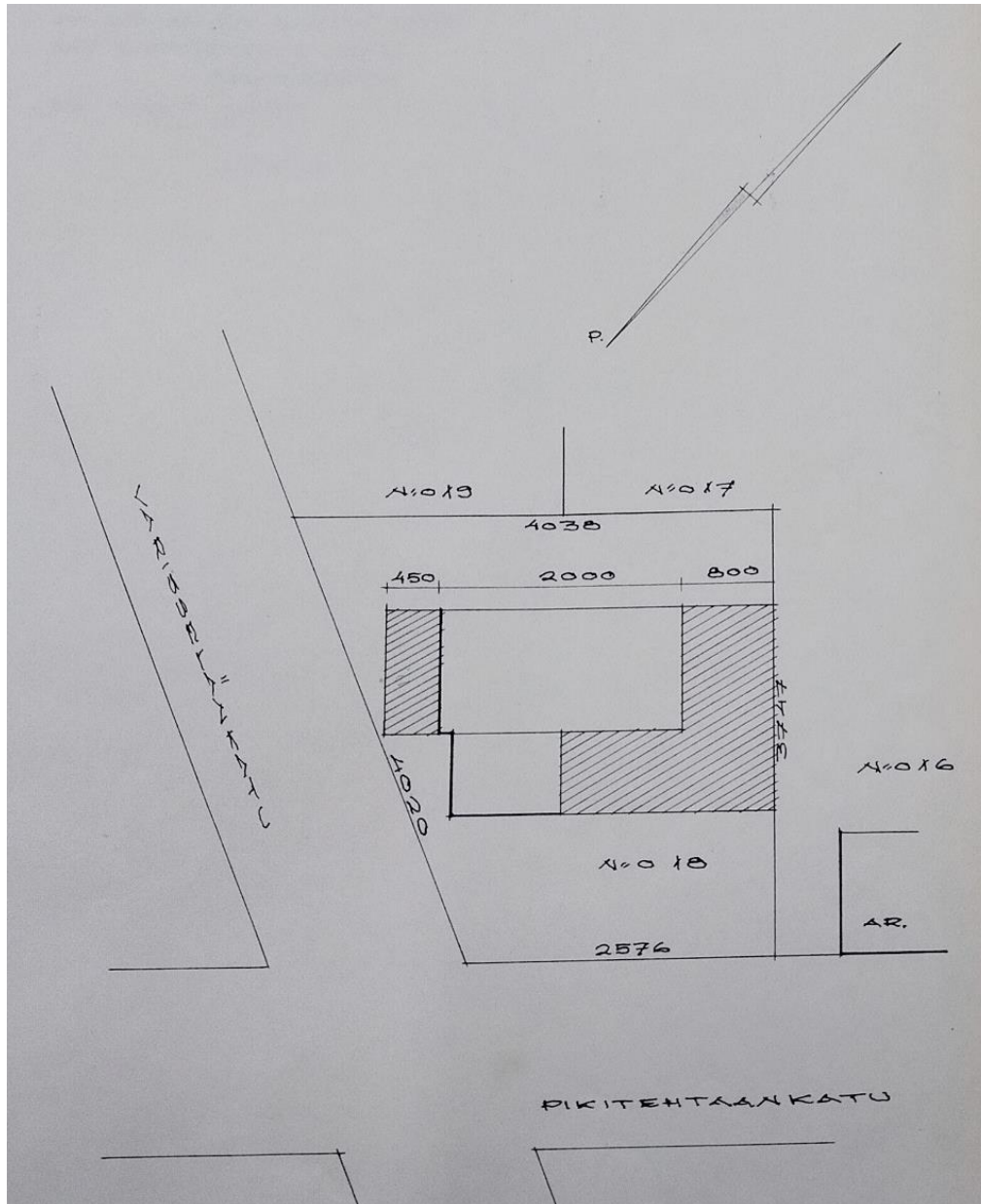
Kuva 27 Asemapiirros 1970-luvun alusta, Vaasan rakennusvalvonnan arkisto
