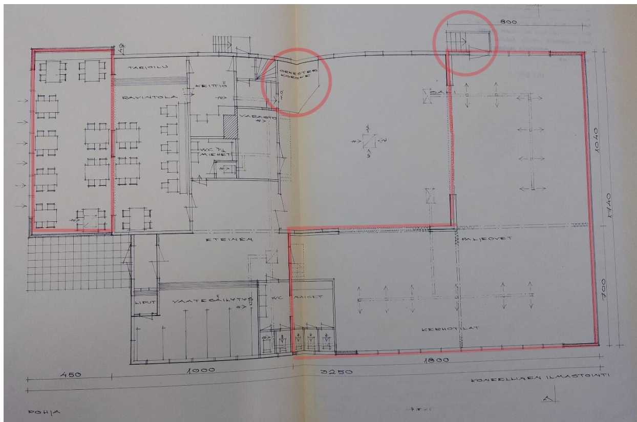
Kuva 29 Pohjakuva työväentalon 1. kerroksesta, laajennusosat ja muutokset merkitty punaisella, Vaasan rakennusvalvonnan arkisto (muokattu 2021)
