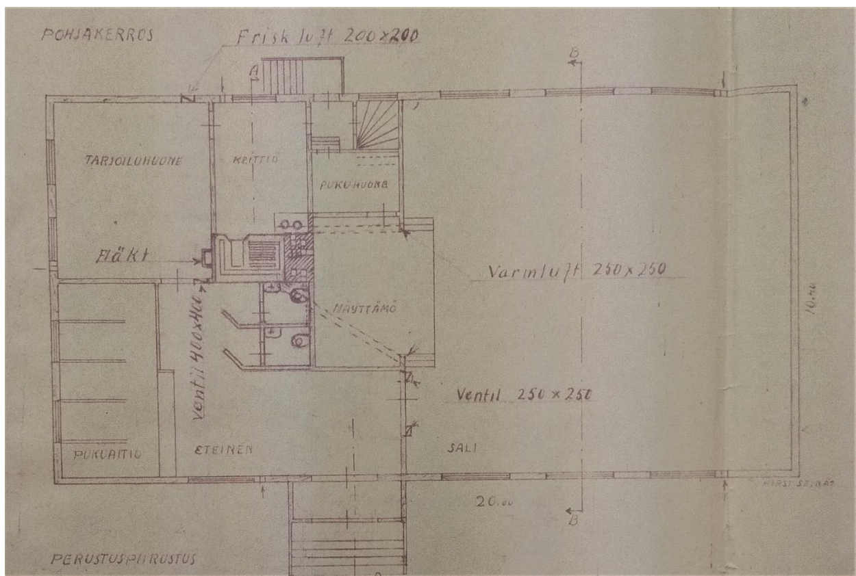
Kuva 18 Emil Nabb, 1948, pohjakerros, Vaasan rakennusvalvonnan arkisto
