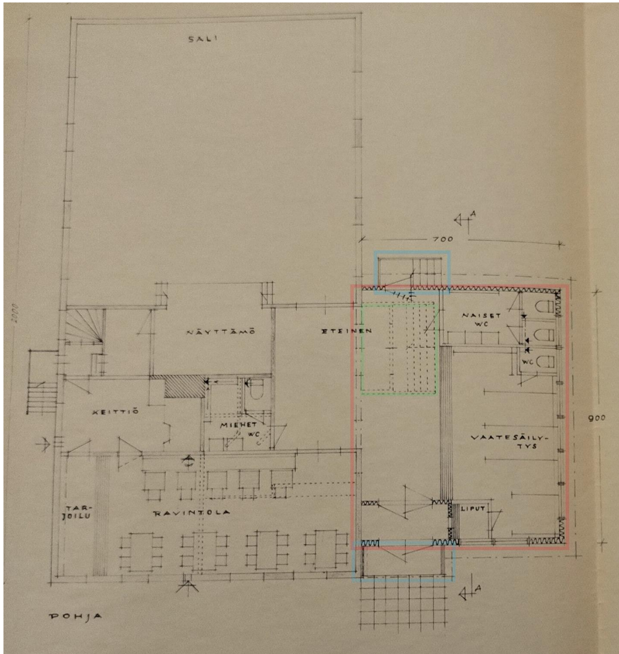
Kuva 26 Vuoden 1964 laajennus, Vaasan rakennusvalvonta (muokattu)
