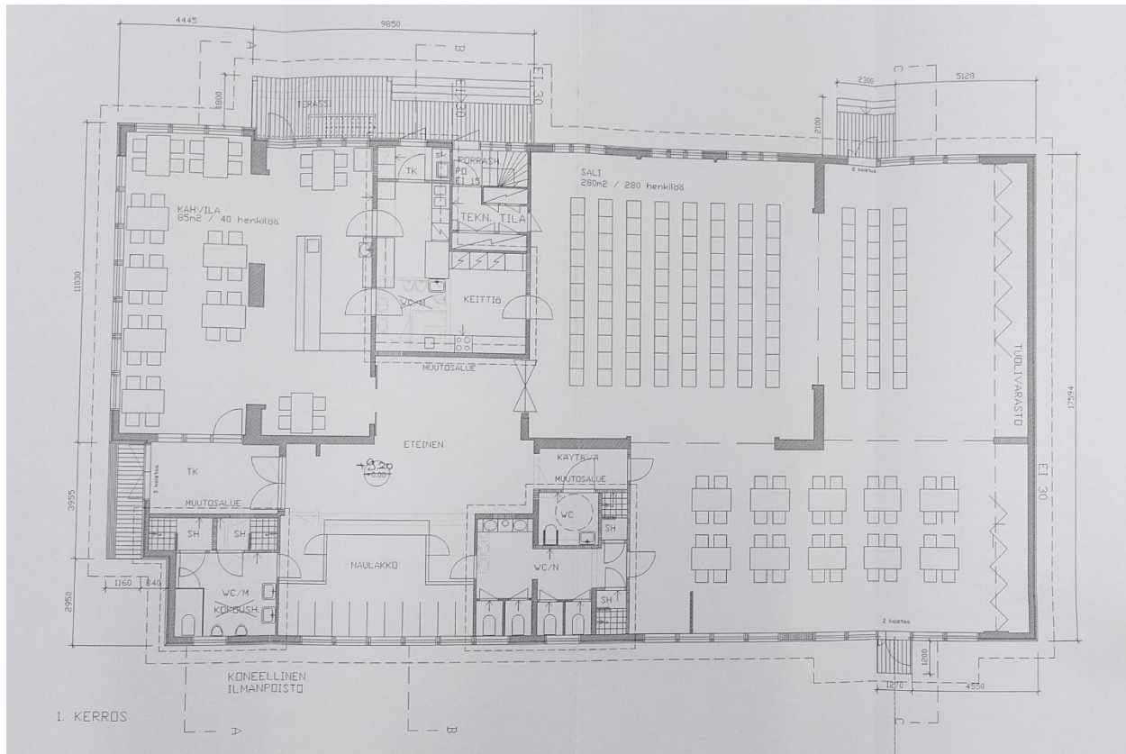
Kuva 31 Waltermannin muutospiirustukset vuodelta 2002, 1. kerros, Vaasan kaupungin rakennusvalvonta
