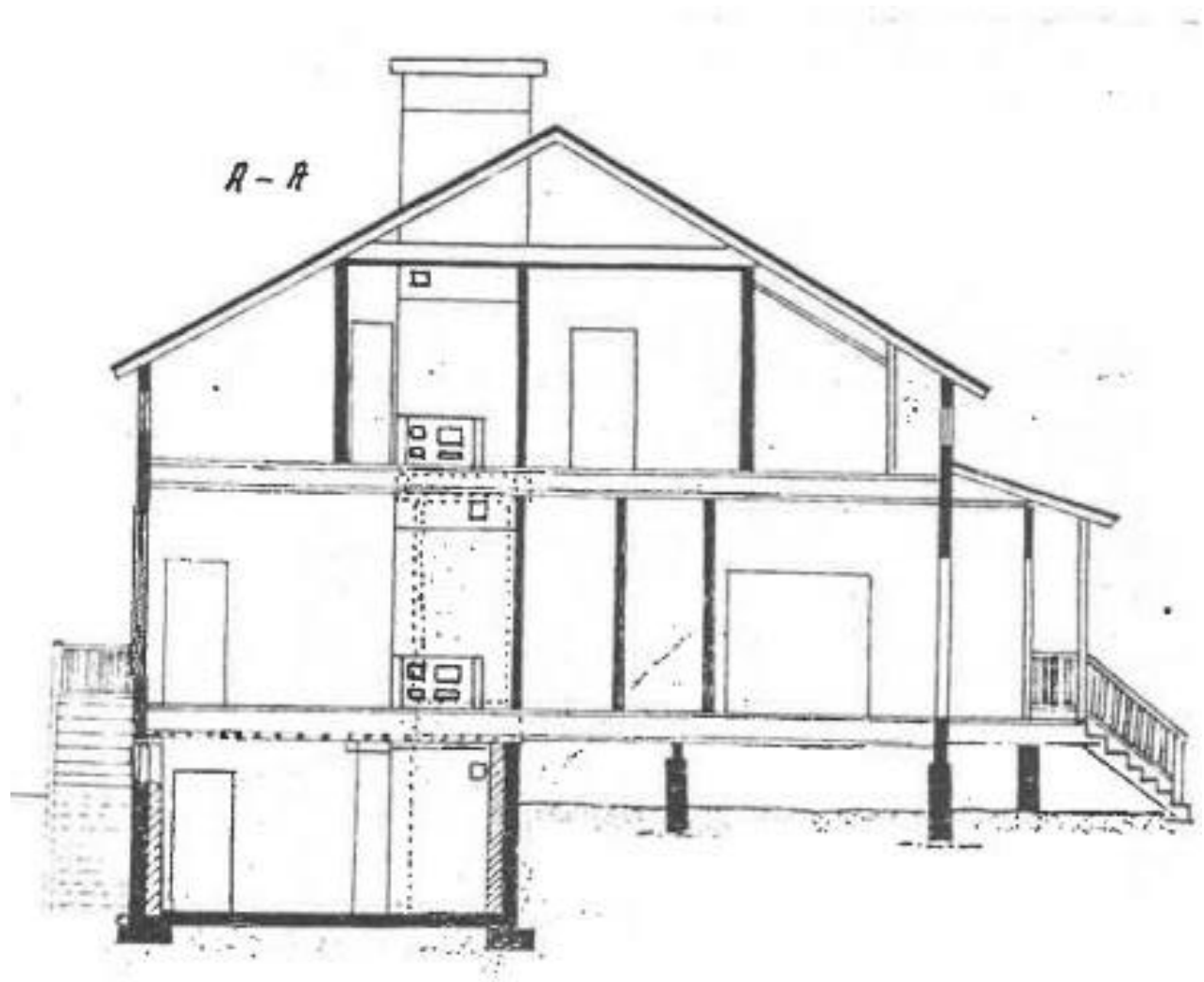
Kuva 21 Ote A. Smulterin piirustuksista Varisselänkadun puolelta, Inventointikortti, Museovirasto
