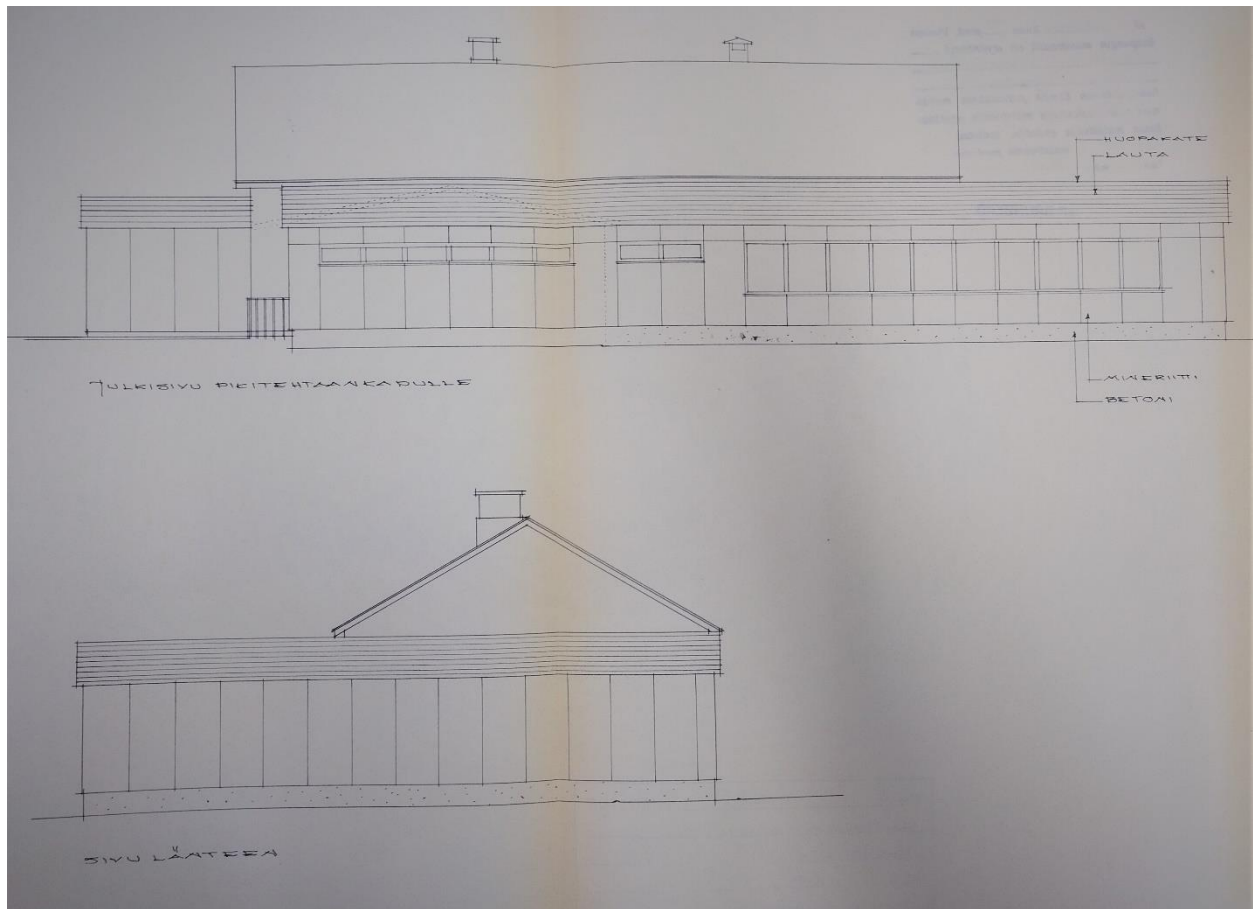
Kuva 28 Julkisivukuvat toisesta laajennusurakasta, Vaasan rakennusvalvonnan arkisto
