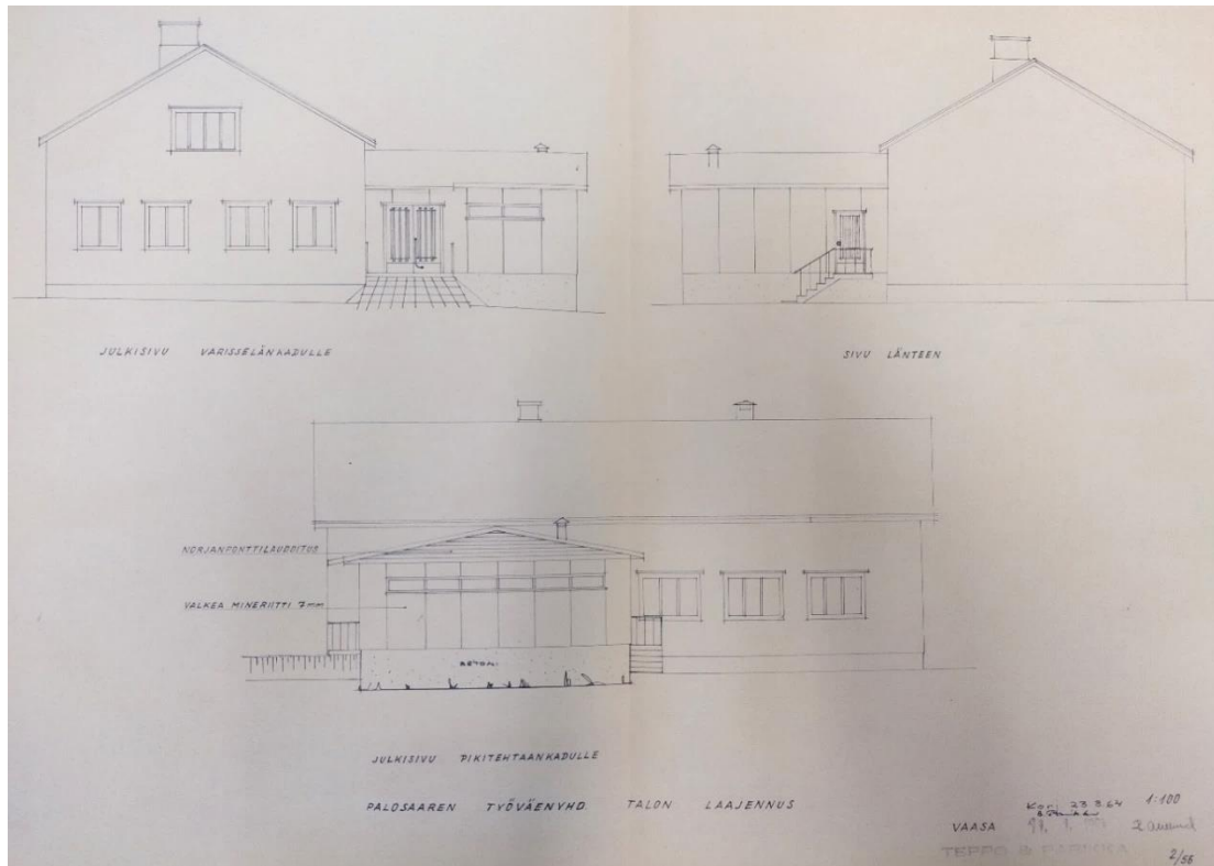
Kuva 24 Julkisivupiirustukset vuodelta 1964, Vaasan rakennusvalvonta
