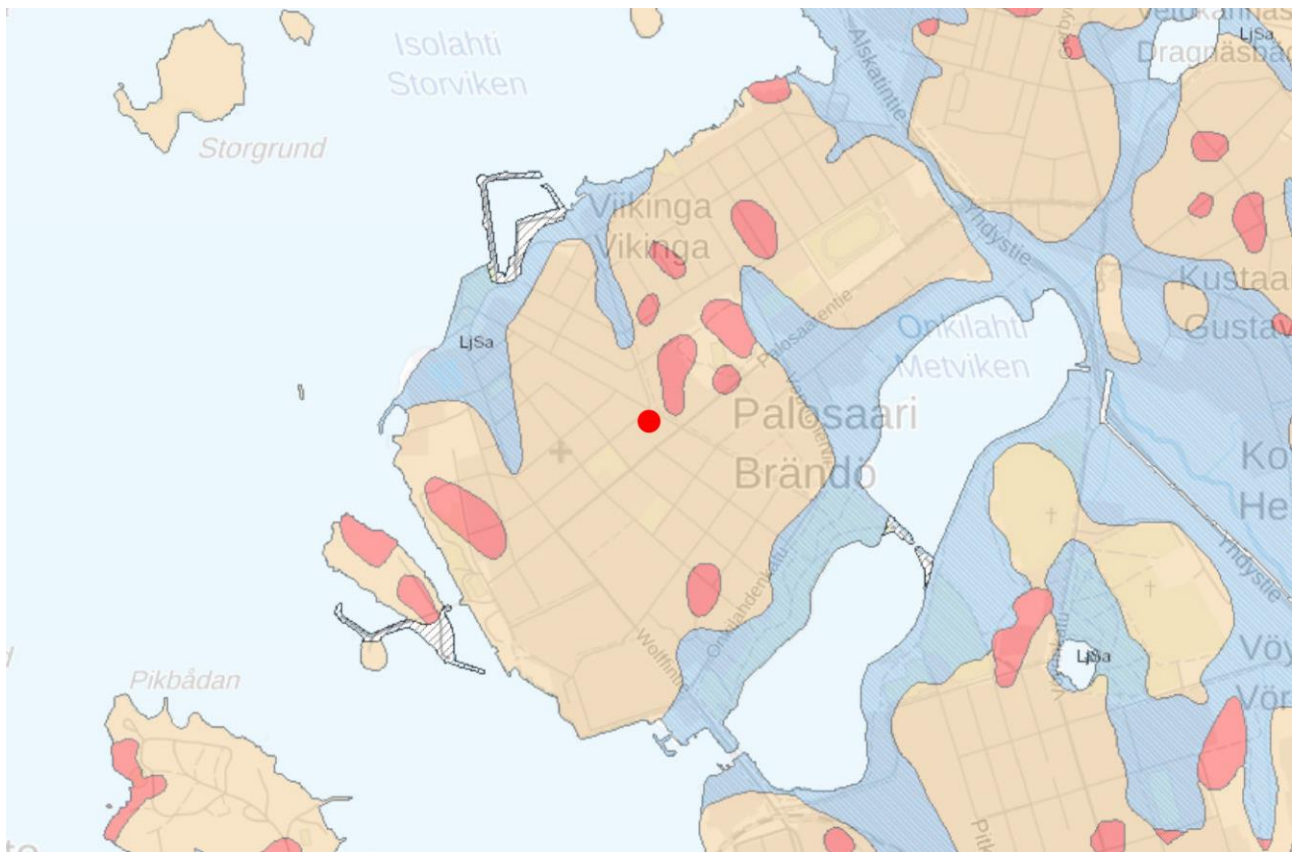
Kuva: Kaavoitusalueen maaperä. Vaaleankeltainen tarkoittaa moreenia, punainen kalliota ja sininen silttisavea. Kaava-alueen likimääräinen sijainti on merkitty punaisella.
