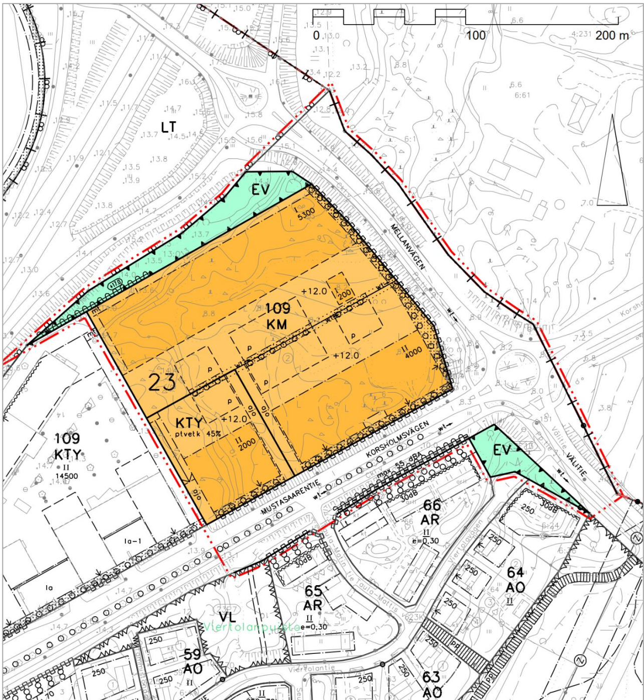
Kivikiilan tarkistus ak1136, asemakaavaluonnos 24.10.2025
