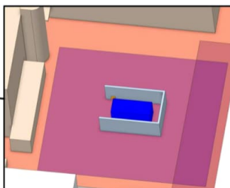
Kuva 14. Vetysäiliön sijoittaminen EnergyLabin tontille siten, että vuoto- ja palorisien vaikutukset kohdistuvat vain omaan tonttiin.
