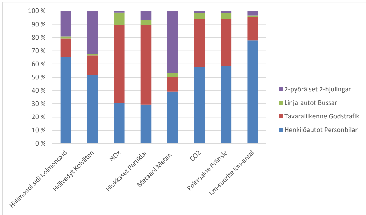
Kuva 4. Eri ajoneuvoryhmien osuus pakokaasupäästöistä, polttoaineen kulutuksesta ja kilometrisuoritteesta yhteisseurannan alueella. Mopopäätöt sisältyvät 2-pyöräisiin. Tavaraliikenne sisältää pakettiautoja ja kuorma-autot.
