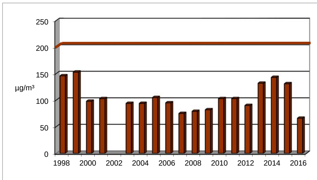
Kuva 20. Raja-arvoon verrannolliset 19. suurimman tunnin typpidioksidipitoisuudet Keskustan mittausasemalla vuosina 1998-2016.
