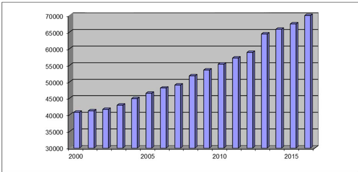
Kuva 2b. Autojen määrä Vaasassa, Mustasaarella ja Maalahdessä vuosina 2000-2016, laskettu Liikenteen turvallisuusviraston tilastoista. Vuosien 2012-2013 eroa selittää Vaasan ja Vähänkyrön kuntaliitos.
