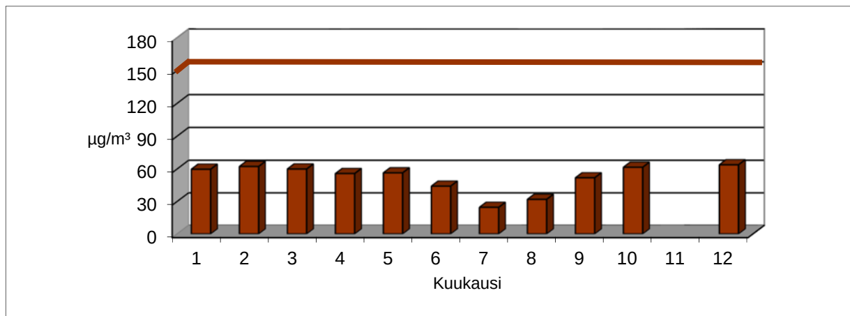
Kuva 8. Typpidioksidipitoisuuksien summafrequenssin 99 % tuntiarvot Vaasassa vuonna 2016. Kuvaan on merkitty ohjearvo (150 µg/m³).
