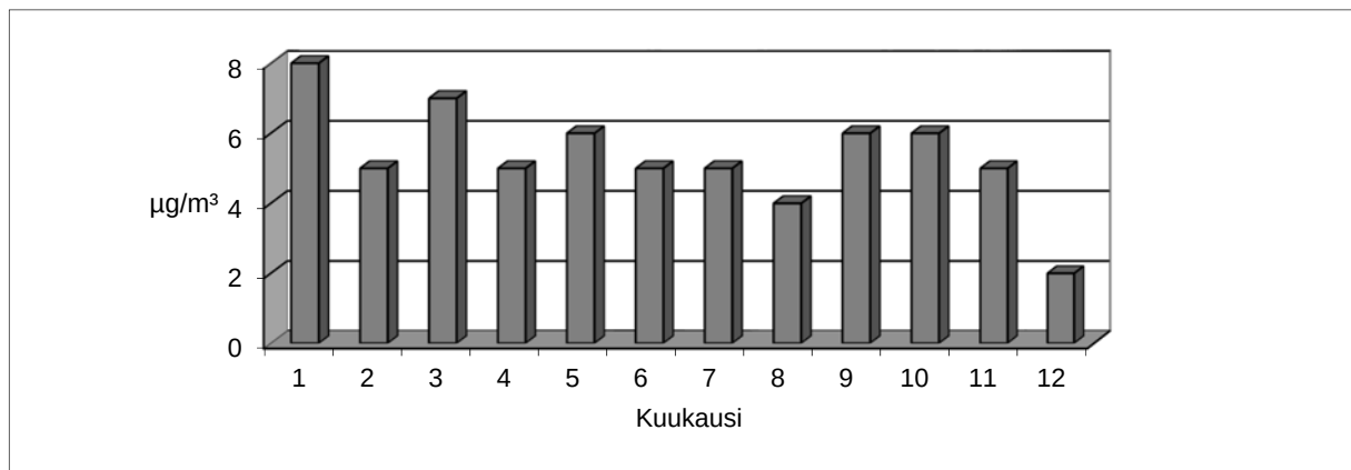
Kuva 15. Pienten hiukkasten kuukausikeskiarvot Vaasassa vuonna 2016.
