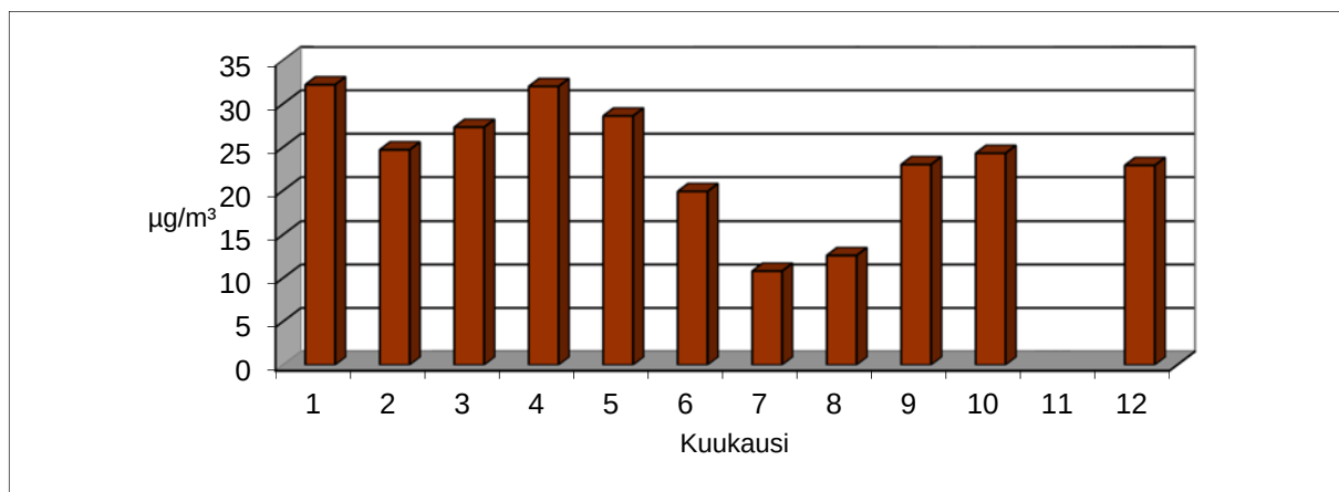
Kuva 6. Typpidioksidin kuukausikeskiarvot Vaasassa vuonna 2016.
