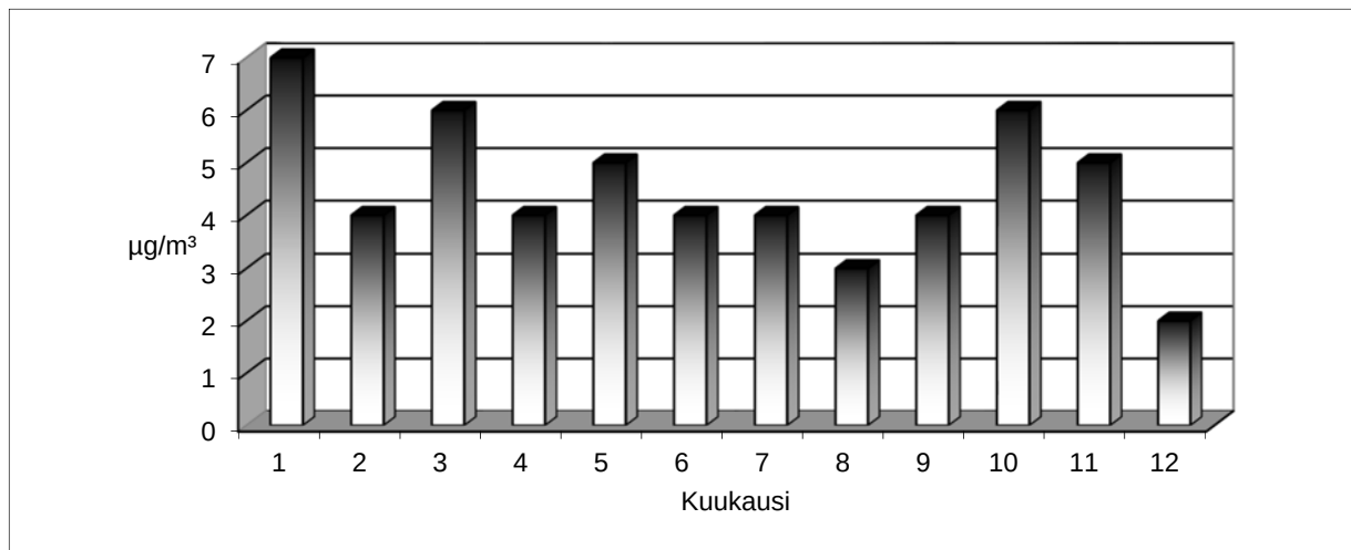
Kuva 18. PM1-hiukkasten kuukausikeskiarvot Vaasassa vuonna 2016.
