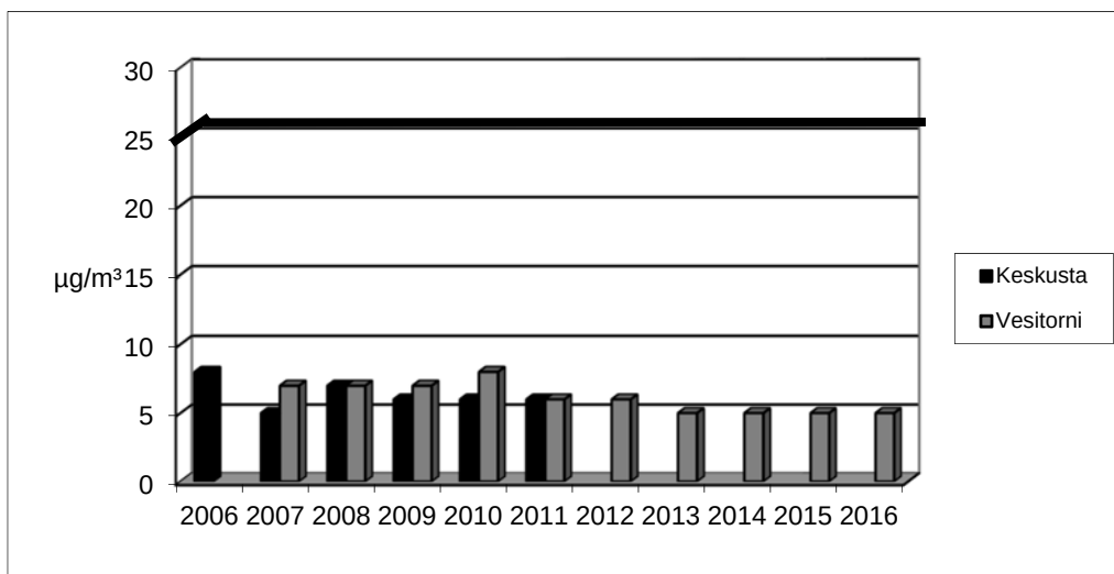
Kuva 25. Raja-arvoon verrannolliset pienhiukkasten vuosikeskiarvopitoisuudet Keskustan mittausasemalla 2006-2011 ja Vesitornin mittausasemalla 2007-2016.
