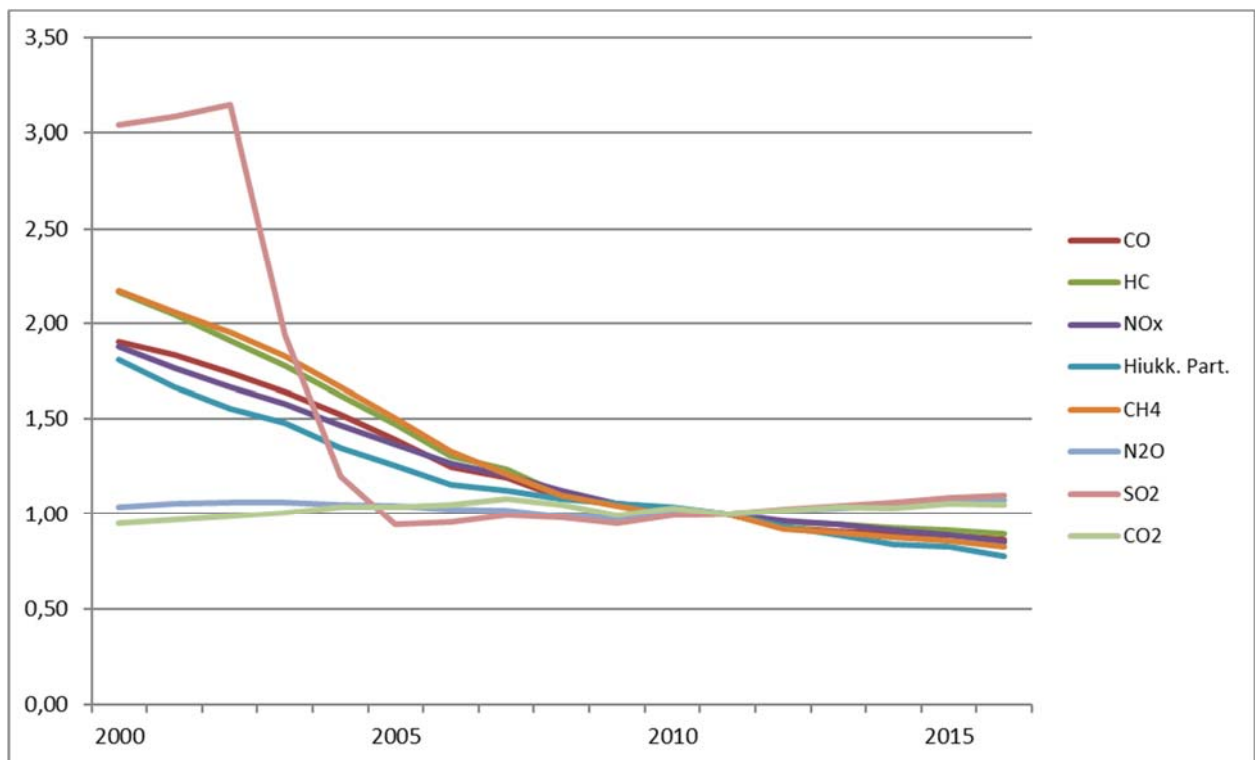
Kuva 2a. Tieliikenteen päästökehitys 2000-2016 (2011=1).
