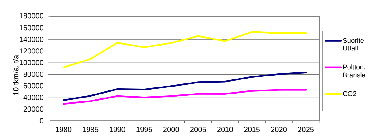
Kuva 3a. Tieliikenteen kilometrisuoritteen, polttoaineenkulutuksen ja hiilidioksidipäästön kehitys ja ennuste Vaasassa, Mustasaarella ja Maalahdessä 1980-2025.
