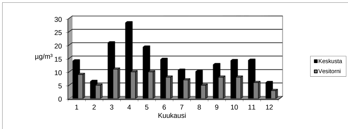
Kuva 13. Hengitettävän pölyn (PM10) kuukausikeskiarvot Vaasassa vuonna 2016.
