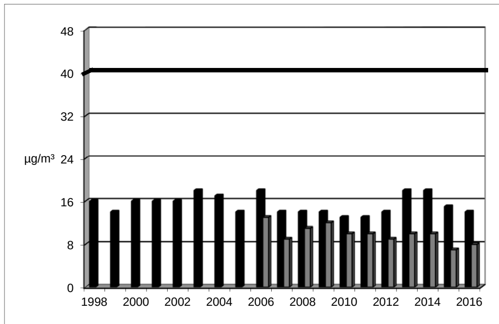
Kuva 24. Raja-arvoon verrannolliset hengitettävien hiukkasten vuosikeski-arvopitoisuudet Keskustan mittausasemalla vuosina 1998-2016 ja Vesitornin mittaus-asemalla 2006-2016.
