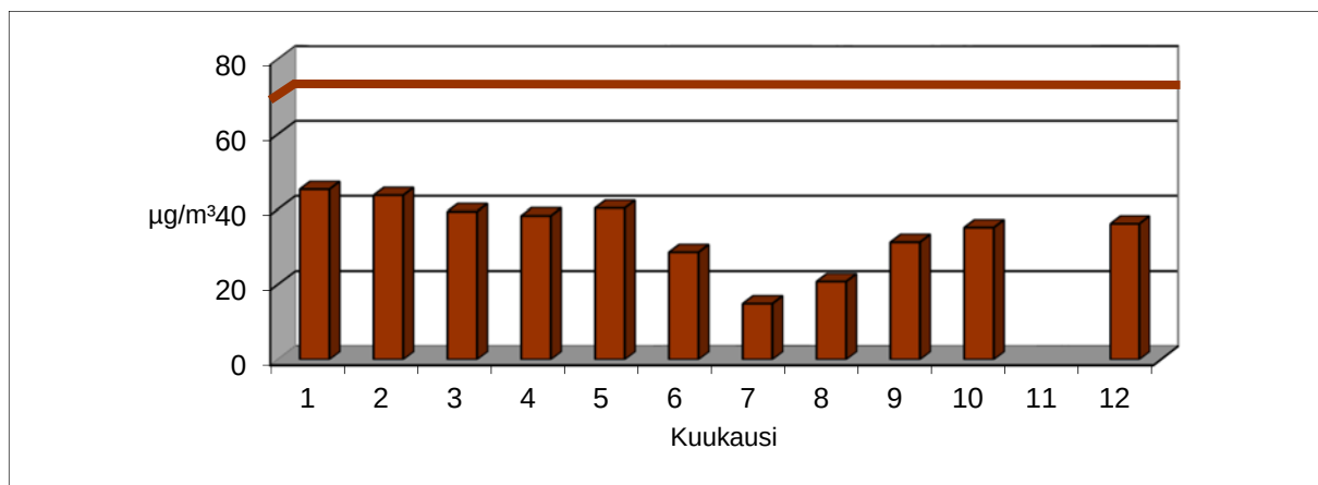
Kuva 7. Typpidioksidin toiseksi suurimmat vuorokausiarvot Vaasassa vuonna 2016. Kuvaan on merkitty ohjearvo ( 70 \mu\text{g}/\text{m}^3 ).
