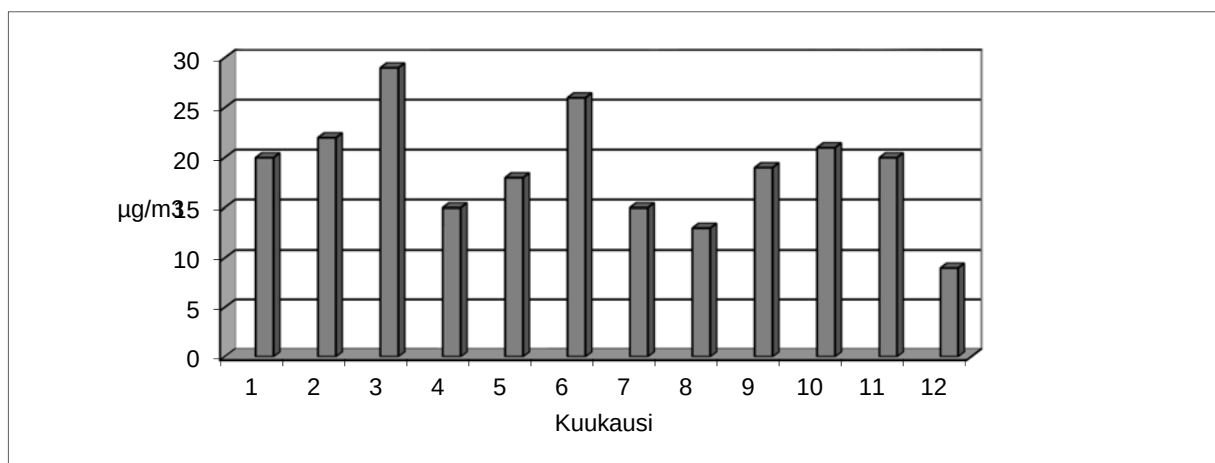
Kuva 17. Pienten hiukkasten suurimmat 8 tunnin arvot kuukausittain Vaasassa 2016.
