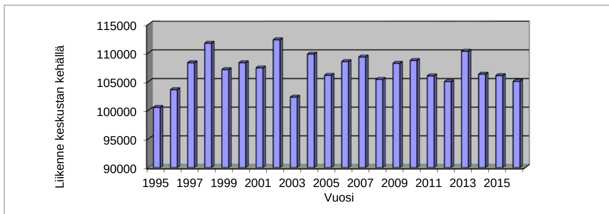
Kuva 1. Vaasan kaupungin liikennesuunnittelun laskemat ajoneuvomäärät keskustan kehällä 1995-2016 (arkivuorokausiliikenne).
