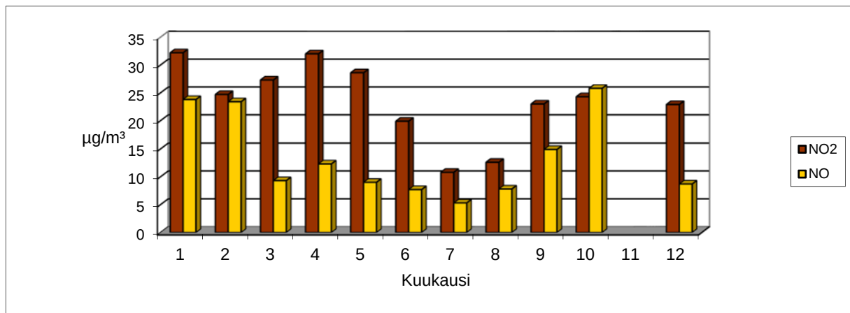
Kuva 9. Typen oksidien kuukausikeskiarvojen vertailu vuonna 2016.
