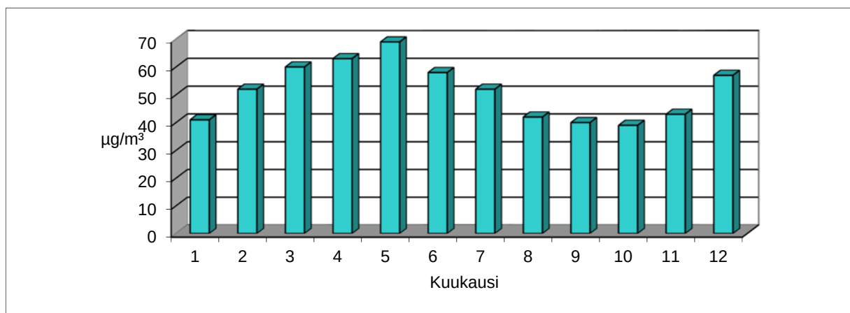
Kuva 10. Otsonipitoisuuden kuukausikeskiarvot Vaasassa vuonna 2016.
