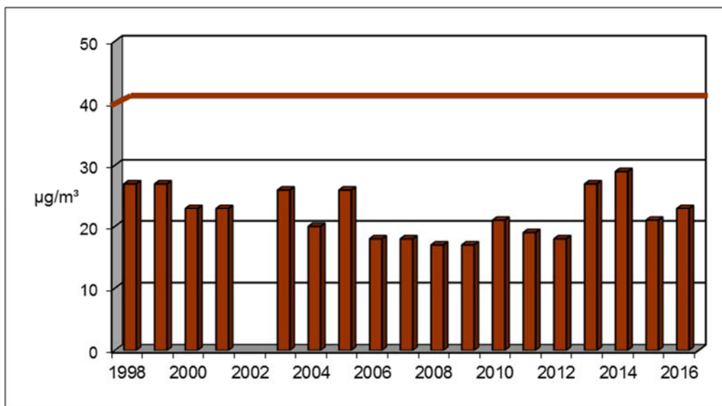
Kuva 21. Raja-arvoon verrannolliset typidioksidin vuosikeskiarvopitoisuudet Keskustan mittausasemalla vuosina 1998-2016.
