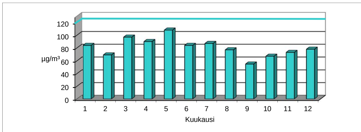
Kuva 11. Otsonipitoisuuden suurimmat 8 tunnin keskiarvot Vaasassa vuonna 2016.
