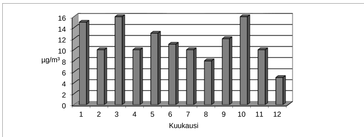
Kuva 16. Pienten hiukkasten toiseksi suurimmat vuorokausikeskiarvot Vaasassa vuonna 2016.
