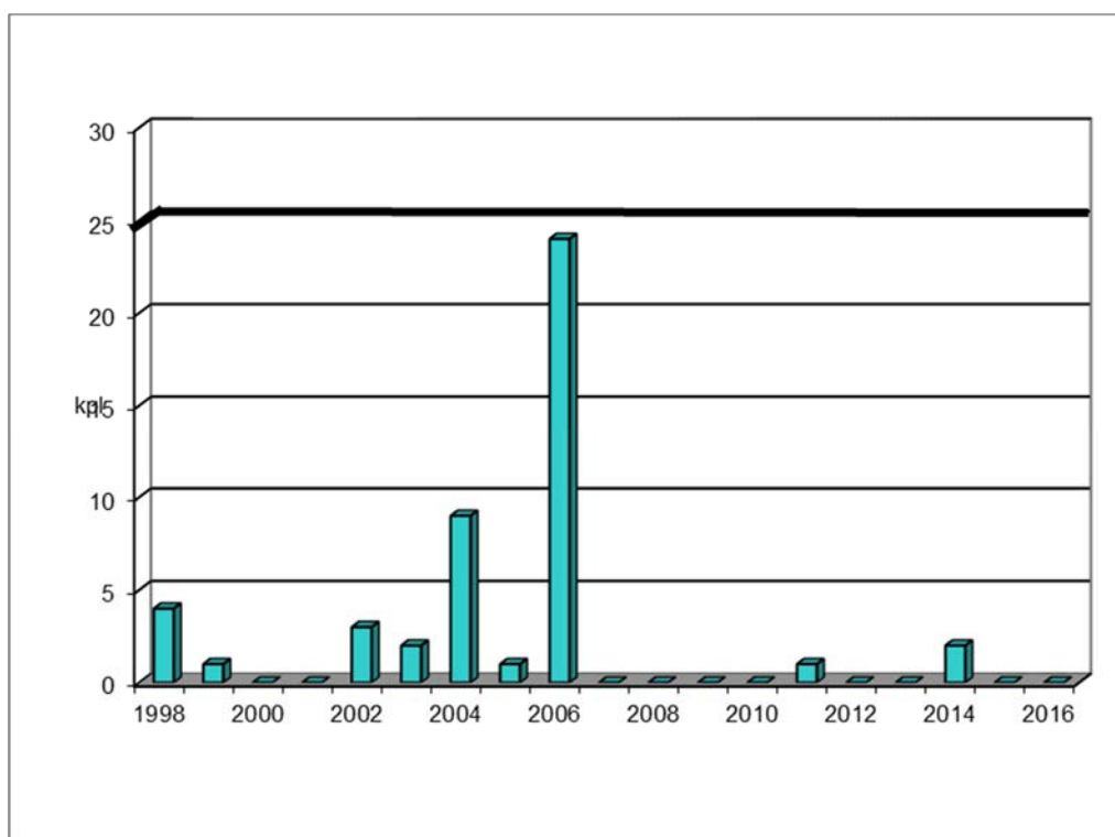
Kuva 22. Otsonipitoisuuden tavoitearvon ylitysvuorokaudet Vaasassa vuosina 1998-2016. Ylityksiä sallitaan 25 kpl vuodessa kolmen vuoden keskiarvona. Mittauspaikka vaihtui vuoden 2005 lopussa.
