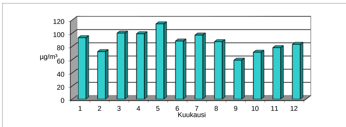
Kuva 12. Otsonipitoisuuden suurimmat tuntiarvot Vaasassa vuonna 2016.
