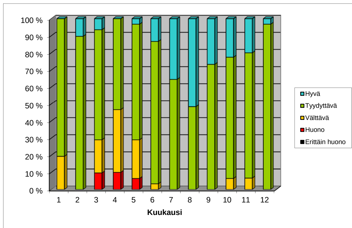
Kuva 19. Ilmanlaatuindeksin päivittäisten arvojen jakautuminen ilmanlaatu luokkiin Vaasassa vuonna 2016.
