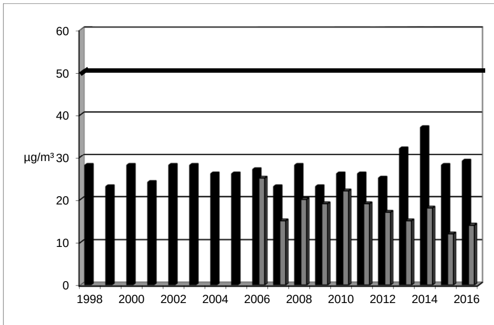
Kuva 23. Raja-arvoon verrannolliset hengitettävien hiukkasten 36. suurimmat vuorokausipitoisuudet Keskustan mittaus-asemalla vuosina 1998-2016 ja Vesitornin mittausasemalla 2006-2016.
