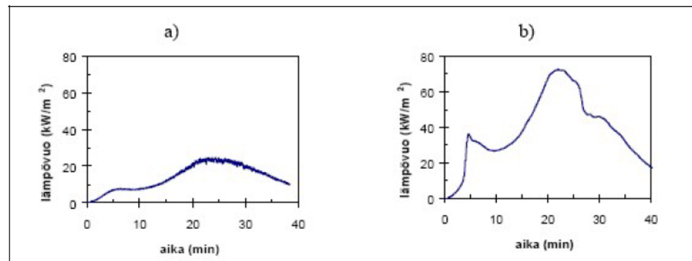
Kuva 6. Autopalon lähistönsä kohdistama lämpösäteily, kun a) auto palaa vapaasti ja b) kun auto palaa katoksessa (LÄHDE: J. Hietaniemi VTT, Tiiviiin ja matalan pientaloalueen paloturvallisuus).
