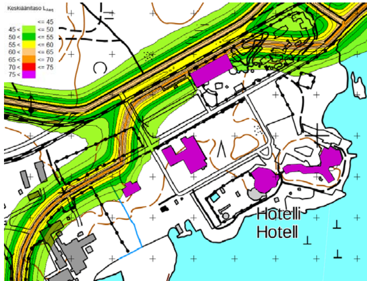
Kuva 20. Yöajan keskiäänitasoalueet 2040 LAeq22-7, putkimallitarkastelu
