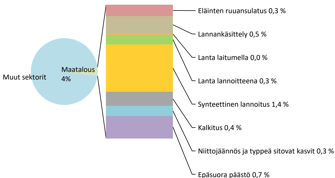
Kuva 9. Maatalouden päästöjen osuus kokonaispäästöistä (ilman teollisuutta) Vaasassa vuonna 2018 ja sektorin jakautuminen eri päästölähteisiin.
