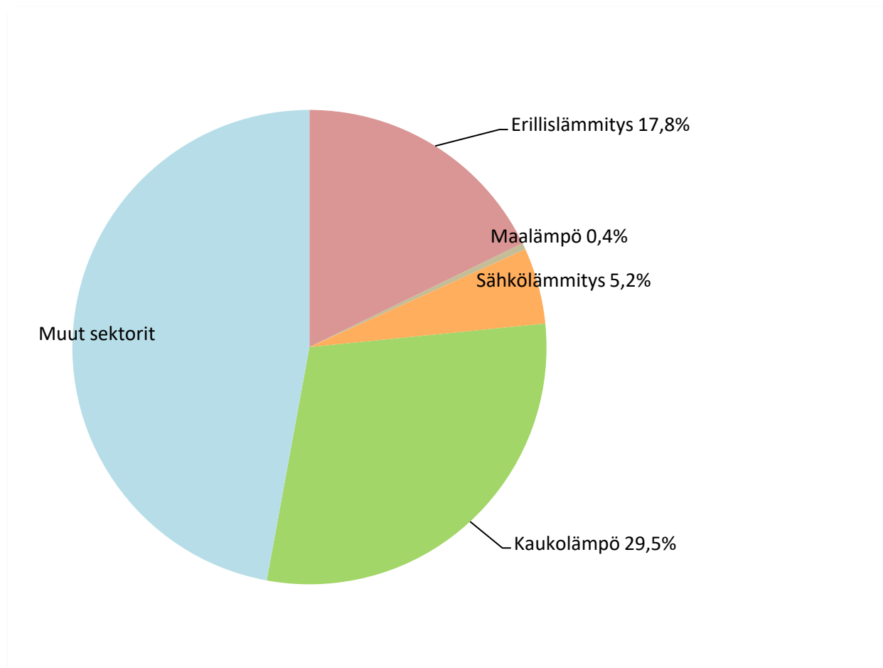
Kuva 5. Rakennusten lämmityksen päästöjen osuus kokonaispäästöistä (ilman teollisuutta) Vaasassa vuonna 2018 ja sektorin jakautuminen eri päästölähteisiin.
