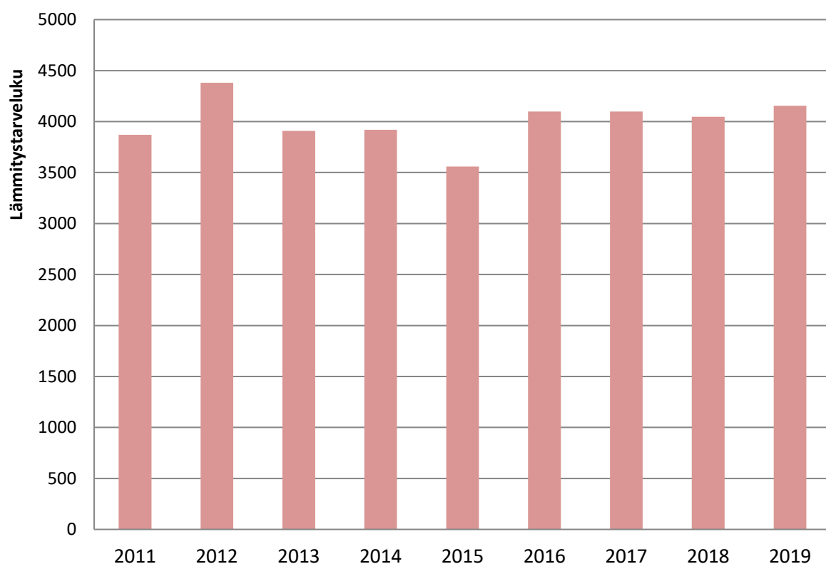
Kuva 4. Vaasan lämmitystarveluvut vuosina 2011–2019.
