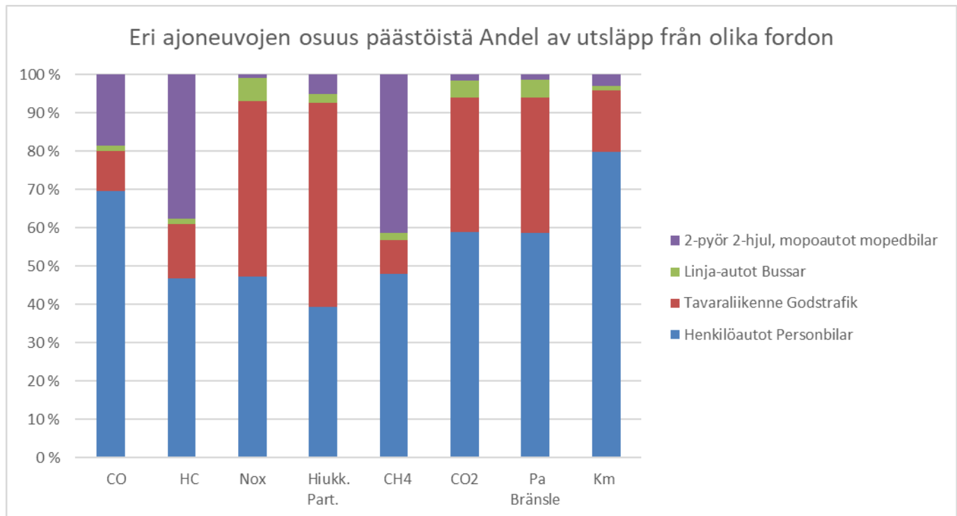
Kuva 4. Eri ajoneuvoryhmien osuus pakokaasupäästöistä, polttoaineen kulutuksesta ja kilometrisuoritteesta yhteisseurannan alueella. Mopoautot sisältyvät 2-pyöräisiin. Tavaraliikenne sisältää pakettiautot ja kuorma-autot.
