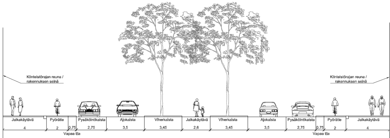
Kuva 41. Puistikoiden tyyppipoikkileikkaus, jossa kulkumuodoille on omat kaistansa, joiden lisäksi pysäköintiä on molemmilla puolilla katua.
