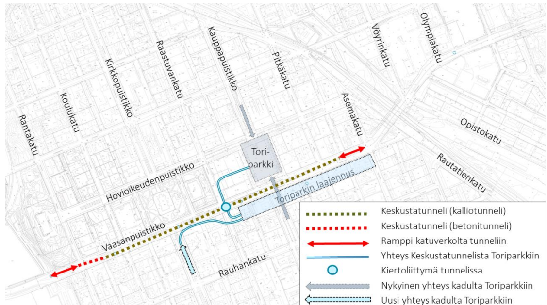
Kuva 20. Keskustatunnelin lyhyt tunnelivaihtoehto
