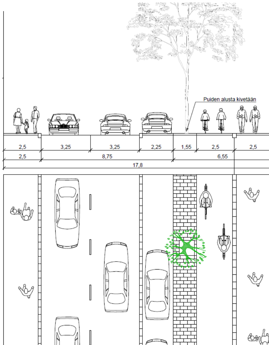
Kuva 39. Pitkälahdenkadun tyyppipoikkileikkaus tavoitetilanteessa. Pyöräilylle lisätään tilaa ja erotellaan jalankulusta. Pysäköinti erotetaan ajoradasta.
