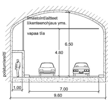
Kalliotunneli kaksi-suuntainen
