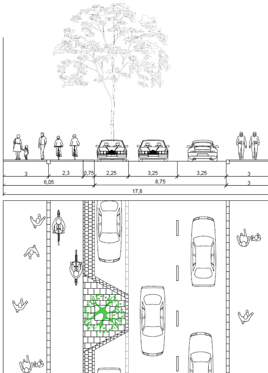
Kuva 40. Pyöräilyn laatukäytän perustyyppipoikkileikkaus esim. Pitkädadulle toteutettuna. Pyöräilylle lisätään tilaa ja erotellaan jalankulusta. Pysäköinti erotetaan ajoradasta puurivin väliin taskuihin.
