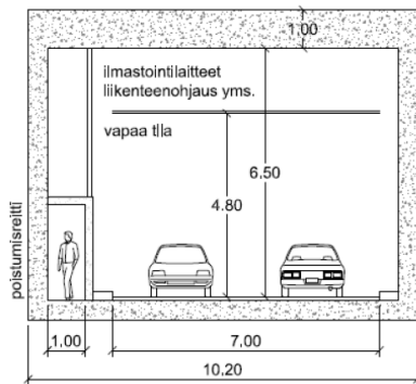
Betonitunneli kaksi-suuntainen
