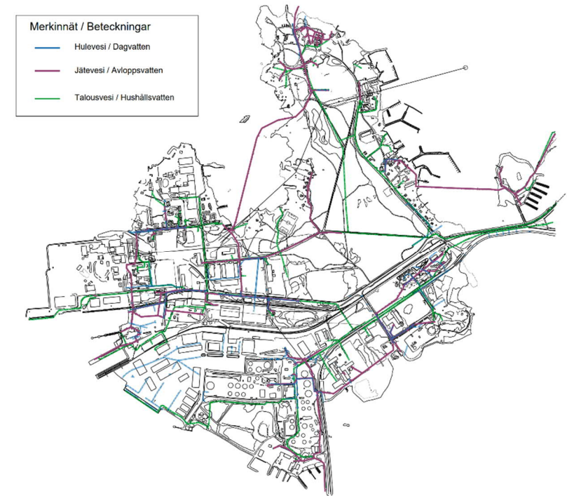
Kuva 38. Vaskiluodon vesihuoltoverkostot.
