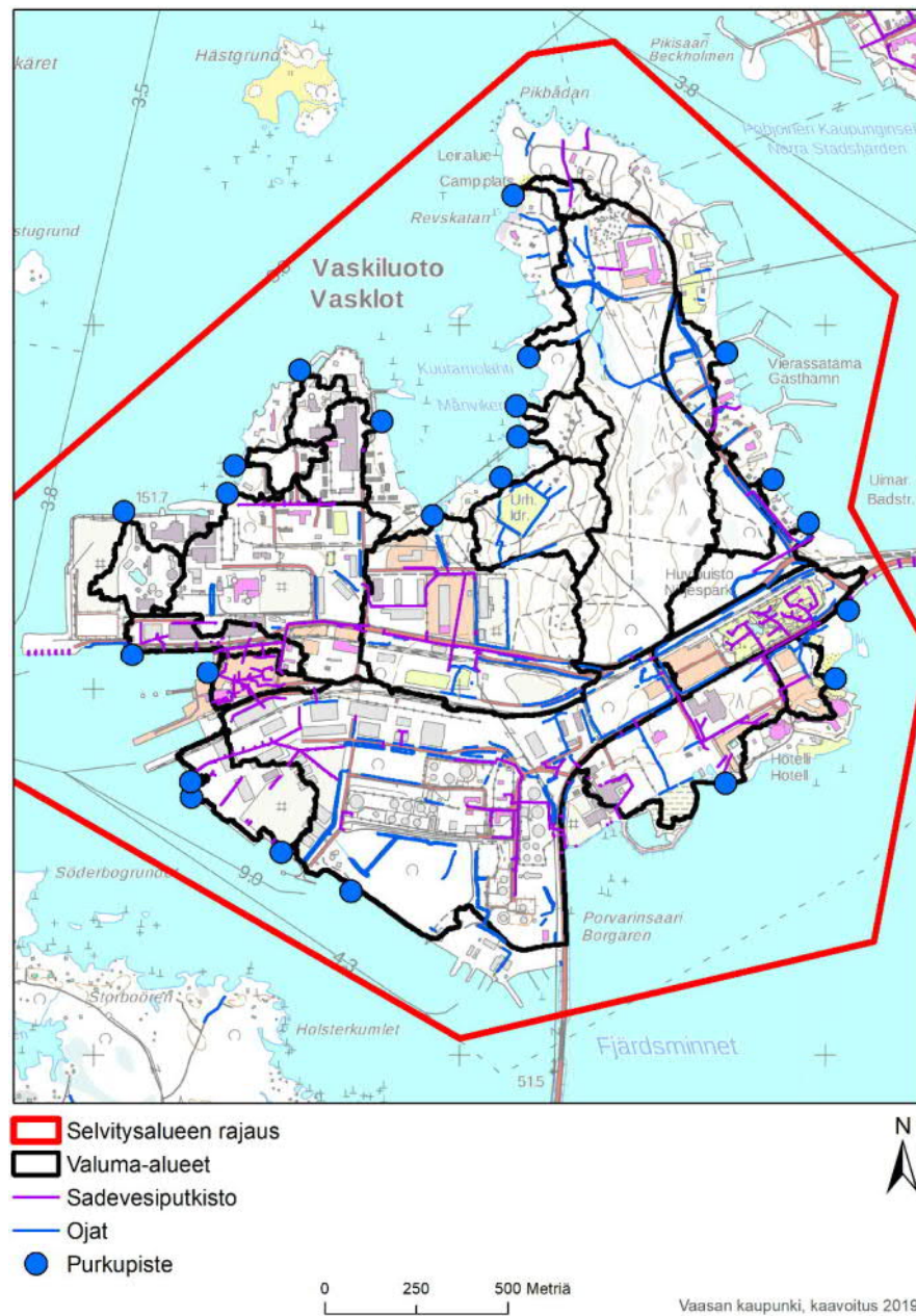
Kuva 33. Selvitysalueen vesiolosuhteet.
