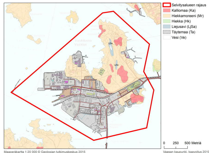
Kuva 36. Alueen maaperäkarta.
