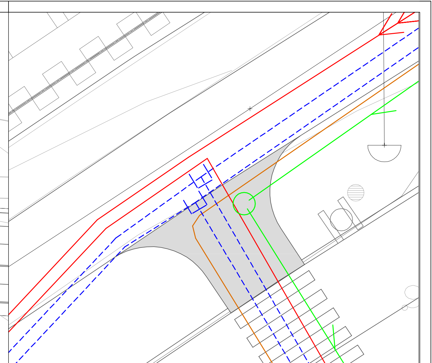
Tuotantotien ja Kivimetsäntien risteyksen putket 1:100
