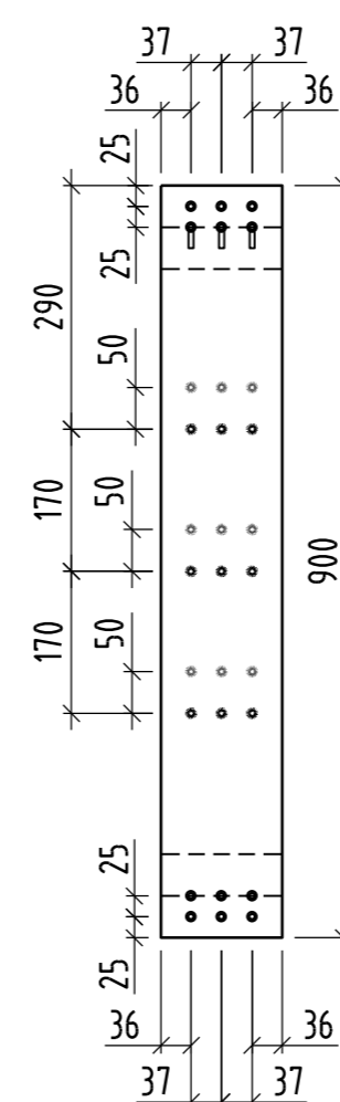
KIINNITYS EDESTÄ 1:10
