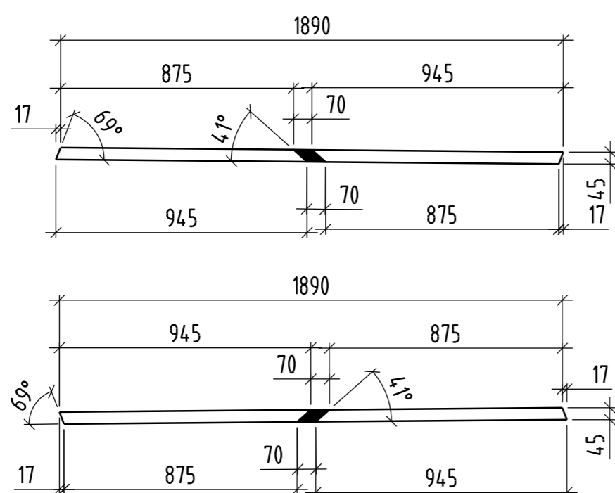
RISTIKON 5 VINOSAUVAT, 1:20
