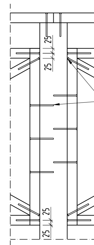
KIINNITYS SIVUSTA 1:10
