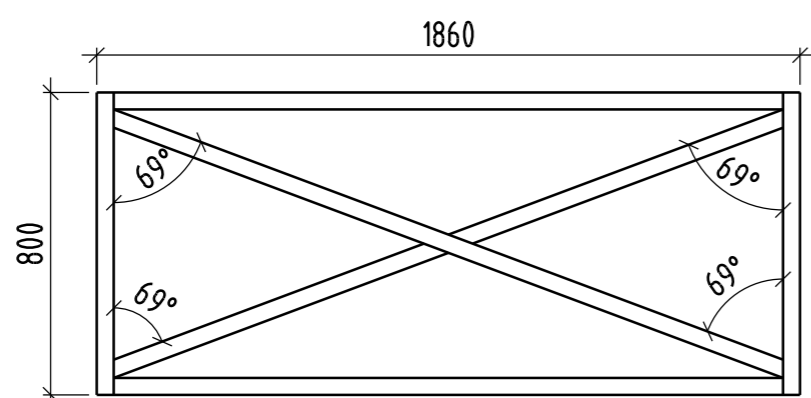
RISTIKON 5 KEHIKKO, 1:20
