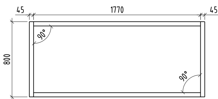
RISTIKON 5 KEHIKKO, 1:20
