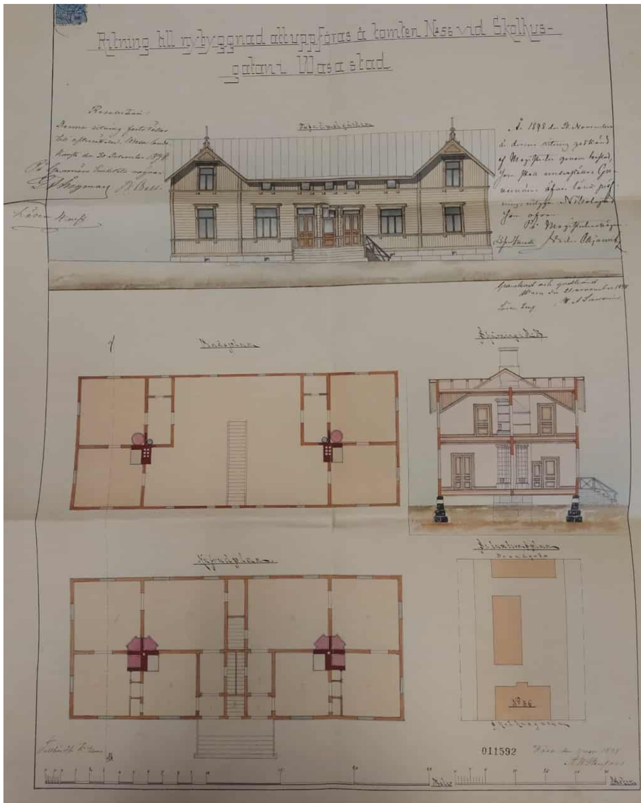
Kuva 21 Alkuperäiset A.W. Stenforsin piirustukset vuodelta 1898, Vaasan kaupungin rakennusvalvonta
