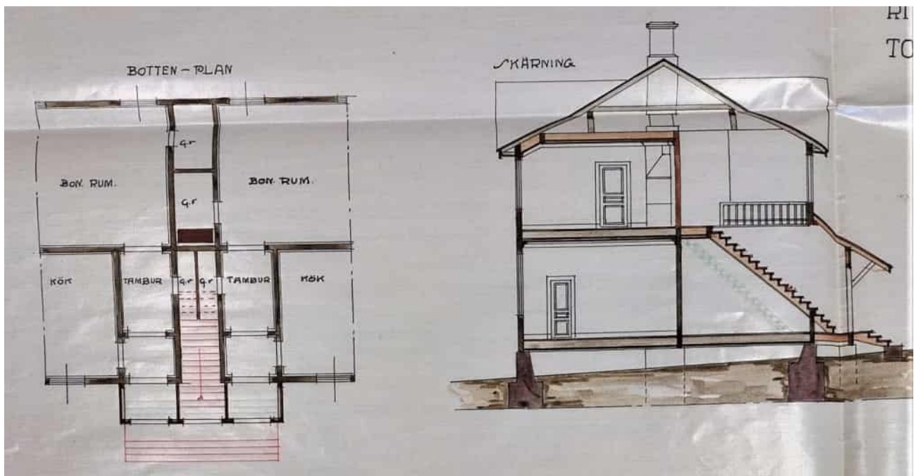
Kuva 22 Vuoden 1923 piirustuksen mukaiset muutostyöt rakennuksen portaisiin, Vaasan kaupungin rakennusvalvonta
