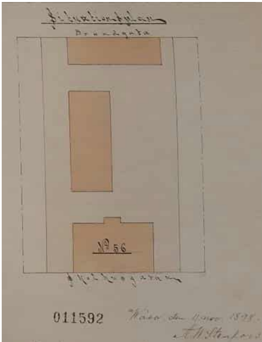
Kuva 42 Vuoden 1898 asemapiirros, A.W. Stenfors, Vaasan kaupungin rakennusvalvonta
