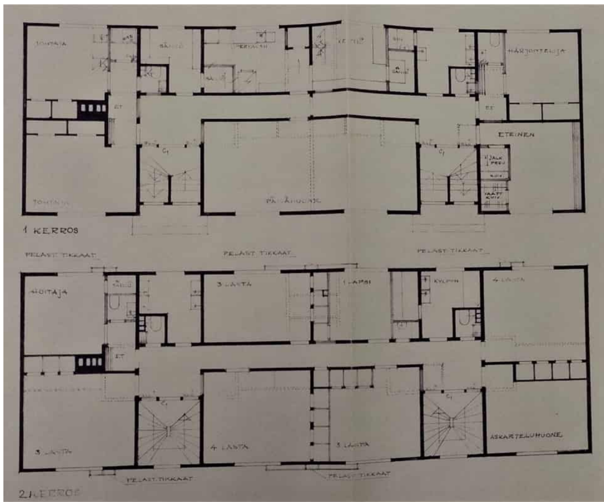
Kuva 36 Sisäiset muutokset vuonna 1960, Vaasan kaupungin rakennusvalvonta
