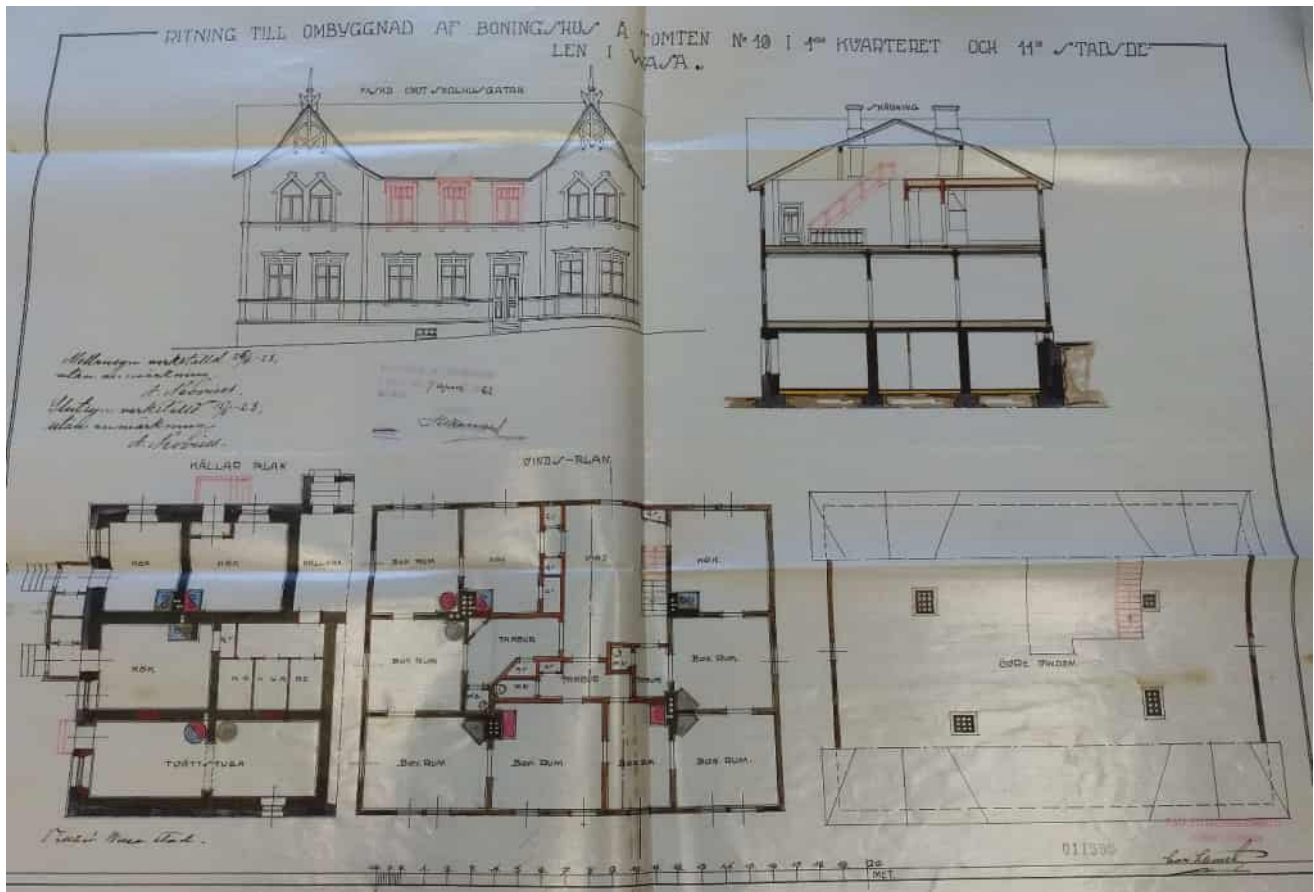
Kuva 7 Carl Schoultzin piirustukset vuodelta 1923, Vaasan kaupungin rakennusvalvonta
