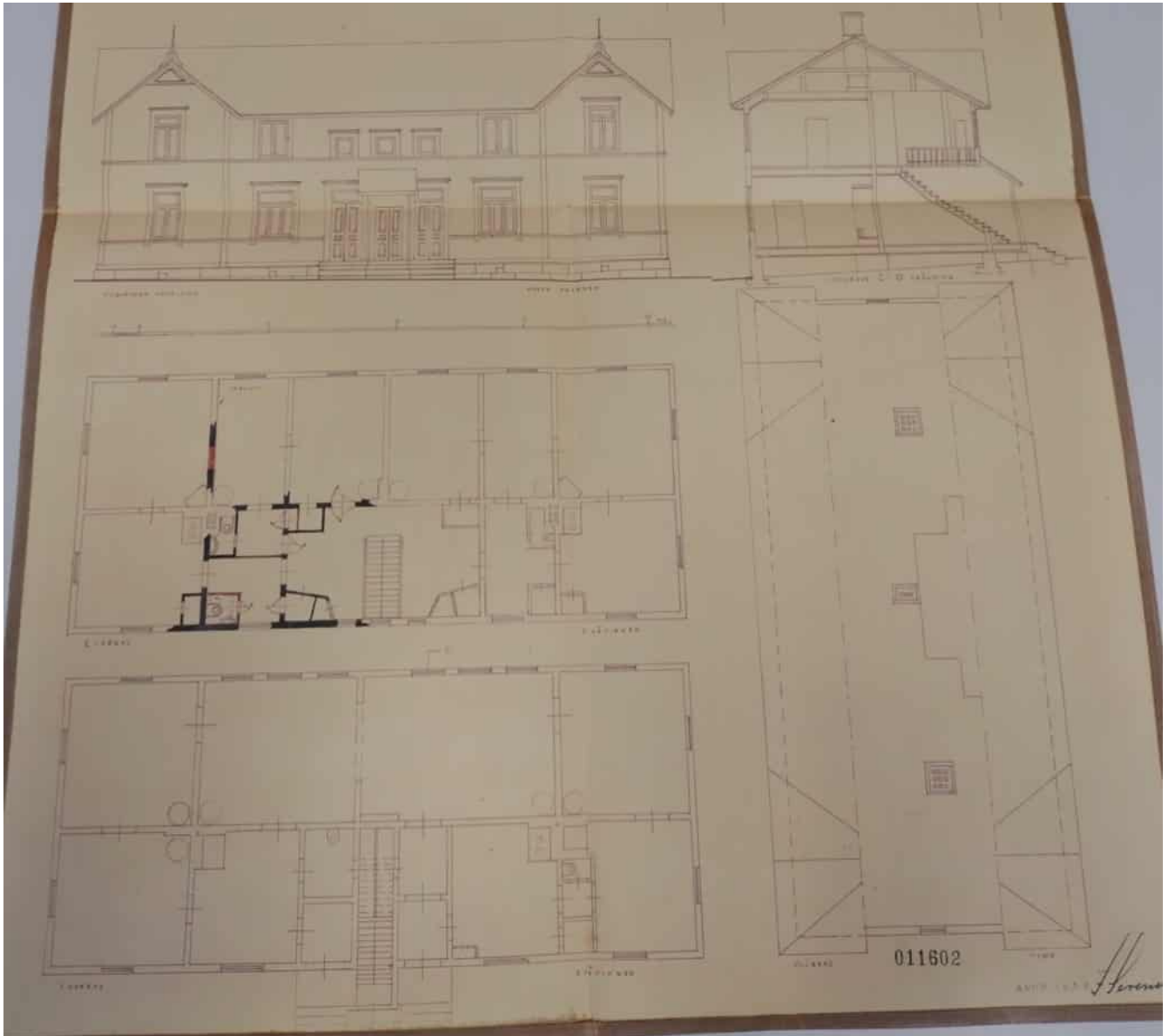
Kuva 23 Vuoden 1938 I. Sereniuksen muutospiirustukset, Vaasan kaupungin rakennusvalvonta
