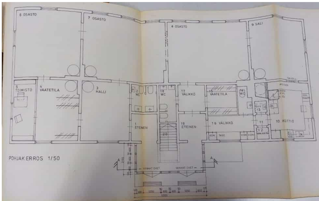
Kuva 25 Kuistimuutos ja 1. kerroksen muutokset, 1984, Vaasan rakennusvalvonnan piirustukset
