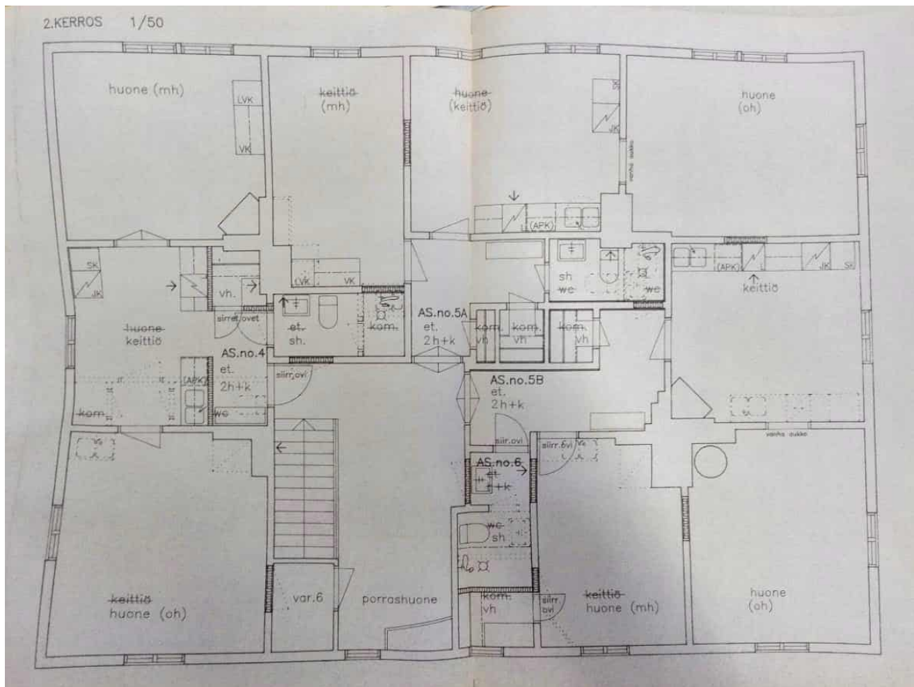
Kuva 13 Viimeisimmät piirustukset sisätiloista vuodelta 1996, 2. kerros, Vaasan kaupungin rakennusvalvonta
