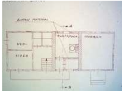
Ulkorakennuksen piirustukset vuodelta 1939. Vaasan kaupungin rakennusvalvonta.
