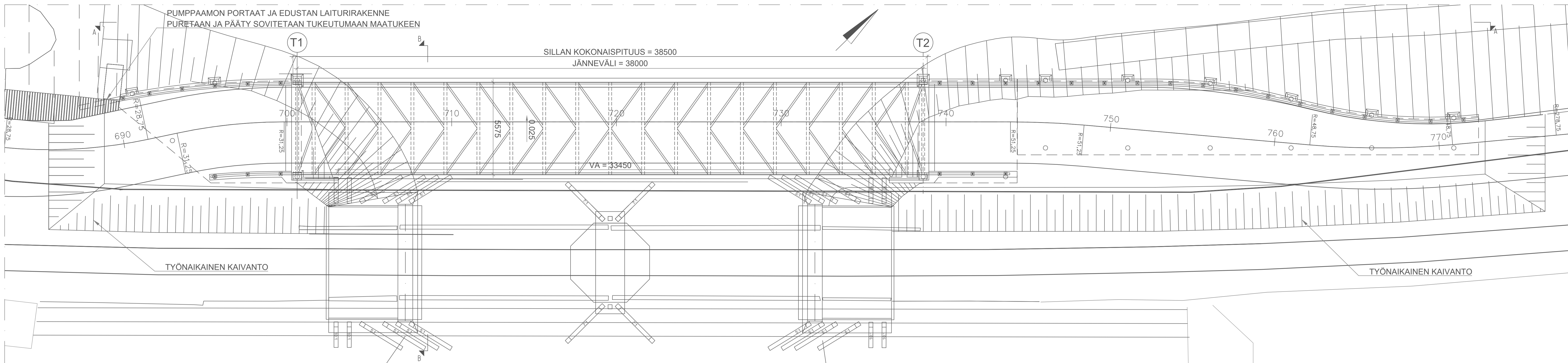
A - A PITUUSLEIKKAUS 1:100
