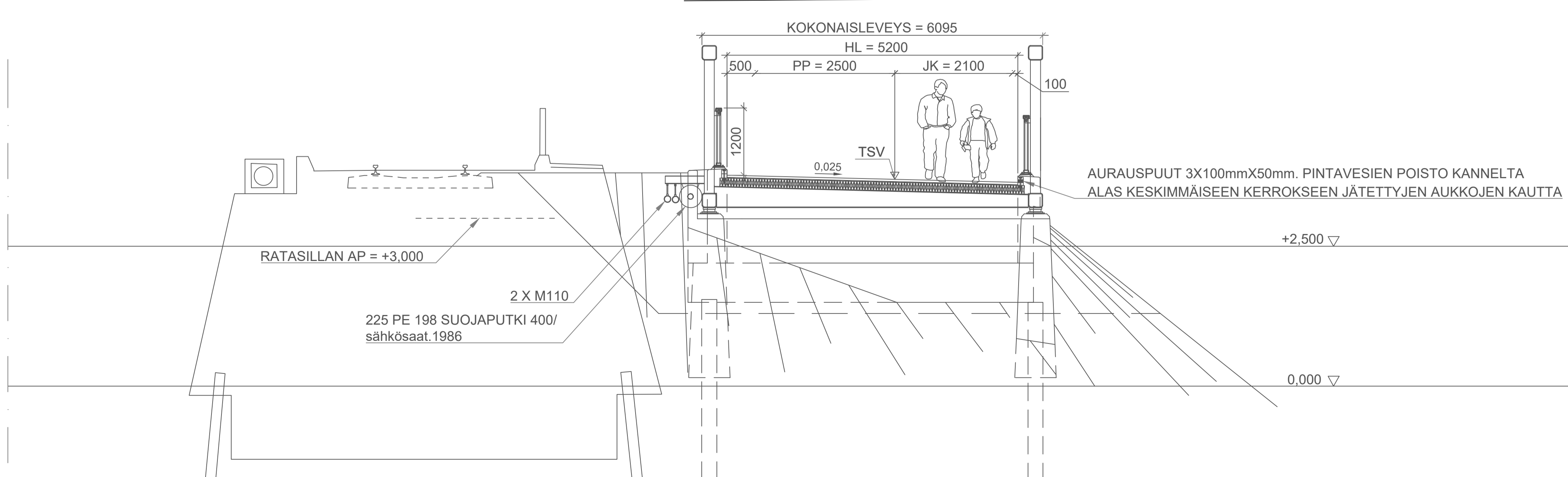
B-B POIKILEIKKAUS MAATUELLA 1:50
